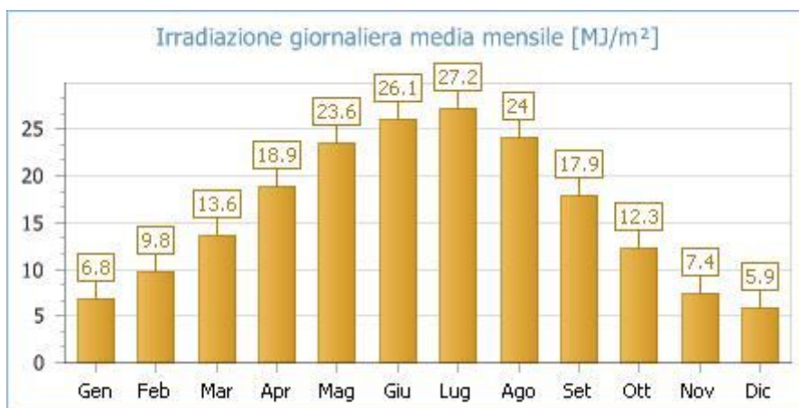
Fig. 2: Irradiazione giornaliera media mensile sul piano orizzontale [MJ/m 2 ]- Fonte dati: UNI 10349 - Località di riferimento: LECCE (LE)/BRINDISI (BR)
